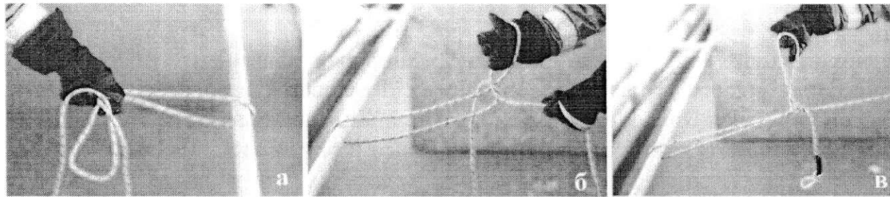
Рис. 1. Закрепление спасательной веревки за конструкцию первым способом
