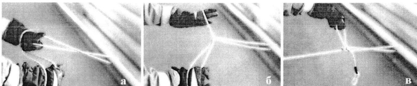
Рис. 3. Закрепление спасательной веревки за конструкцию третьим способом
